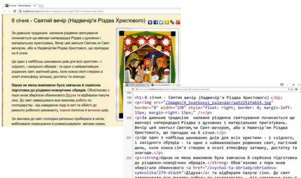
Мал. 9.17. Фрагмент веб-сторінки та відповідний фрагмент HTML-коду
